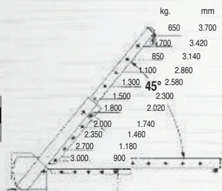
Croquis entrada uñas
